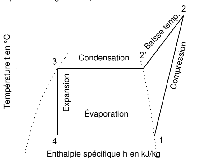
Fig. 2-5. Diagramme t, h d'un cycle du fluide frigorigène
