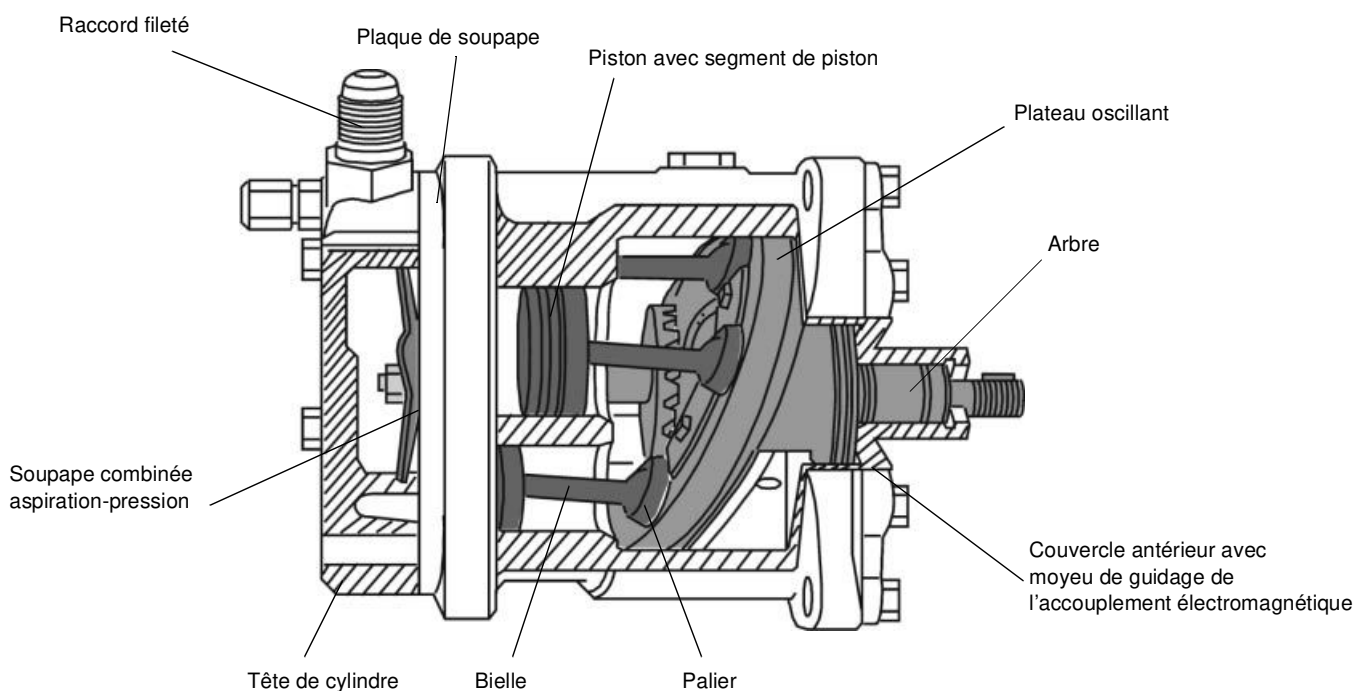
Fig. 4-5. Coupe à travers un compresseur à piston axial
