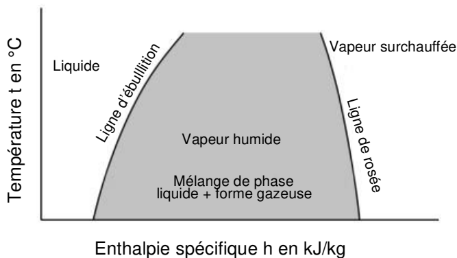
Fig. 2-4. Diagramme t, h
