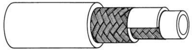
Fig. 4-45. Flexible avec support-pression tressé (2 couches)
