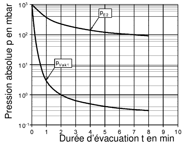
Fig. 7-6. Allure de la pression dans la pompe à vide et dans l'installation
