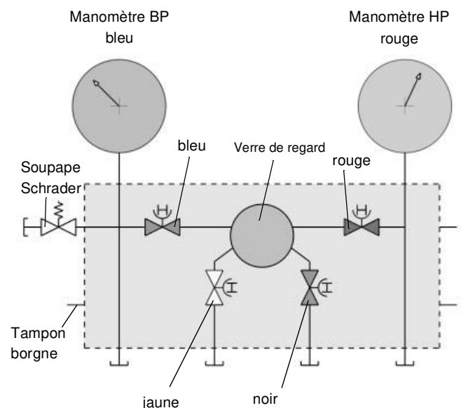
Fig. 7-11. Construction d'un portique de manomètre
