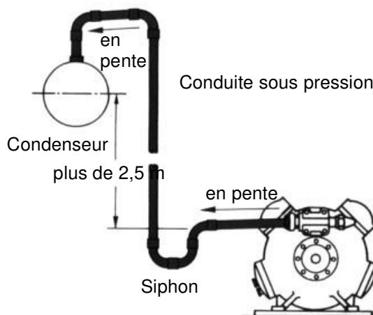
Fig. 4-47. Pose d'une conduite sous pression pour un évaporateur en position élevée
