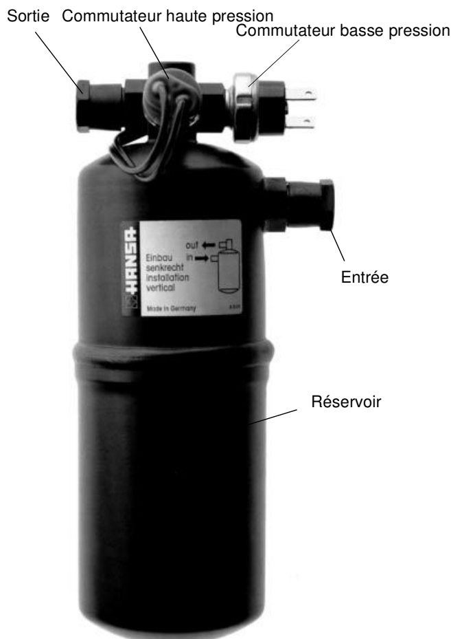
Fig. 4-20. Collecteur d'une installation frigorifique d'automobile
