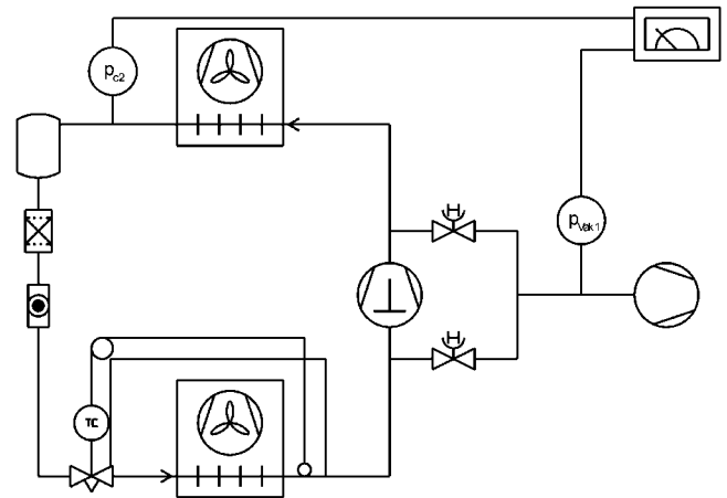
Fig. 7-5. Représentation schématique d'une évacuation bilatérale
