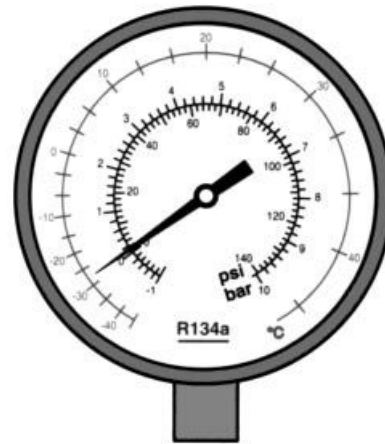
Fig. 1-8. Manomètre avec échelle de températures de saturation
