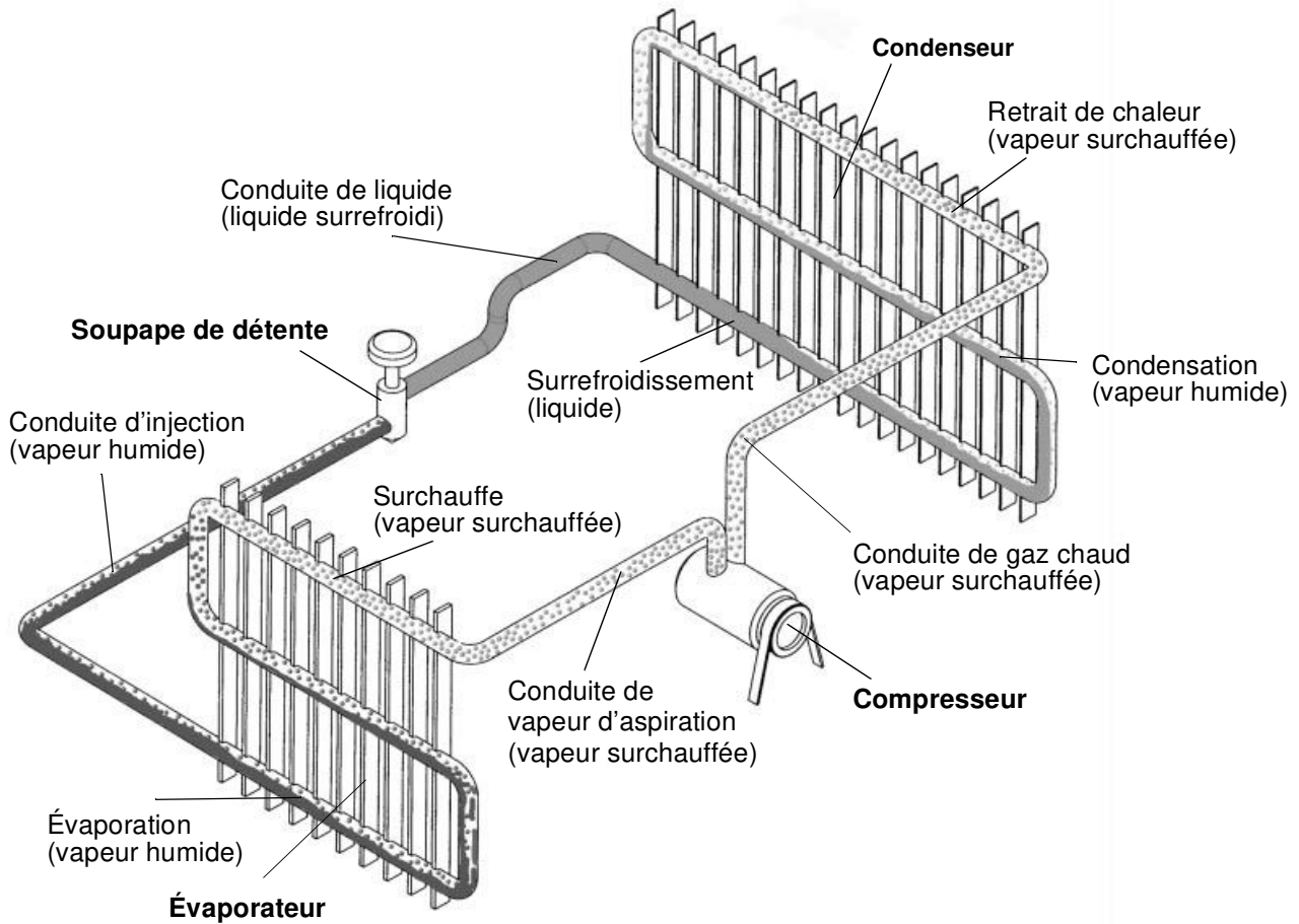
Fig. 2-8. Circuit schématique du fluide frigorigène
