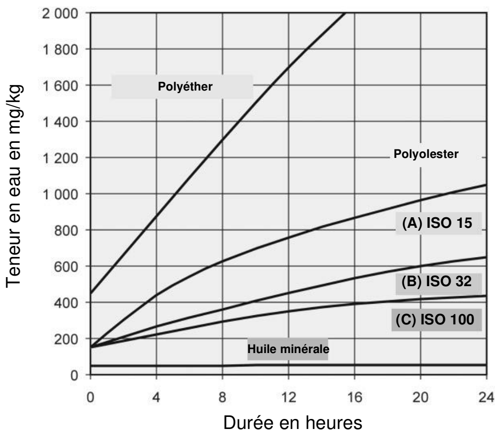
Bild 7-2. Absorption d'eau pour différents types d'huiles
