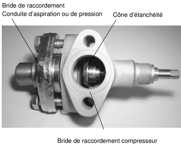
Fig. 7-12. Soupape d'arrêt de compresseur
