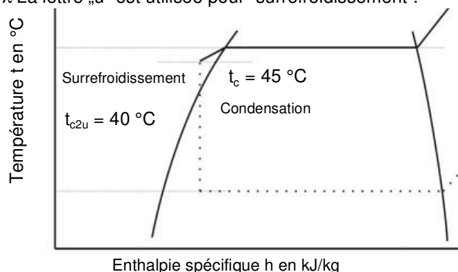
Fig. 2-7. Surrefroidissement du fluide frigorigère
