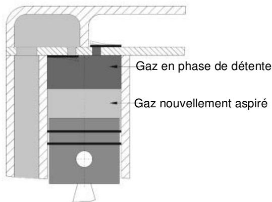
Fig. 3-3. Effet de l'espace nuisible
