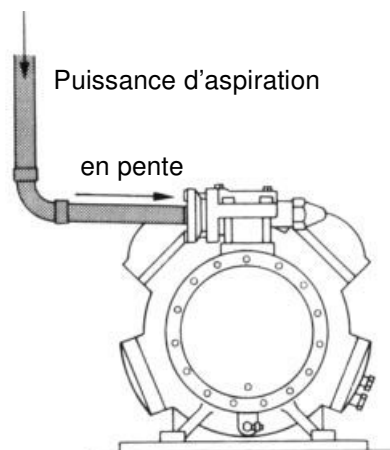
Fig. 4-46. Pose d'une conduite d'aspiration sur le compresseur
