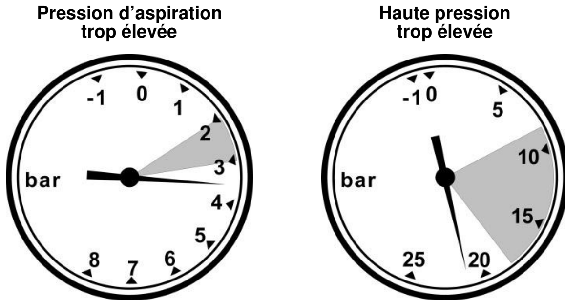
Fig. 8-8. Pression d'aspiration trop élevée, haute pression trop élevée
