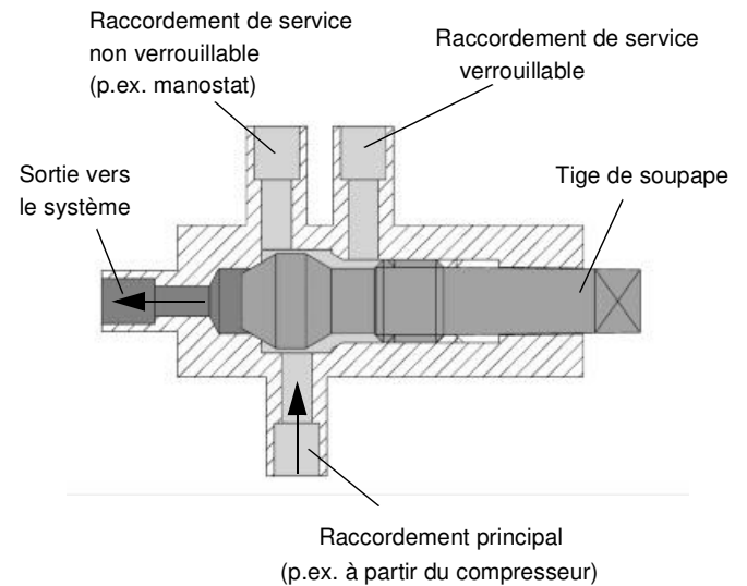
Tige de soupape complètement à gauche, conduite principale fermée
