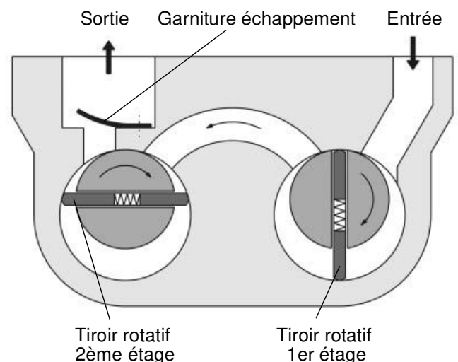
Fig. 7-3. Représentation schématique d'une pompe à tiroirs rotatifs à deux étages
