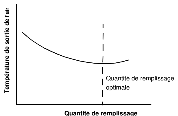
Fig. 7-17. Quantité de remplissage optimale
