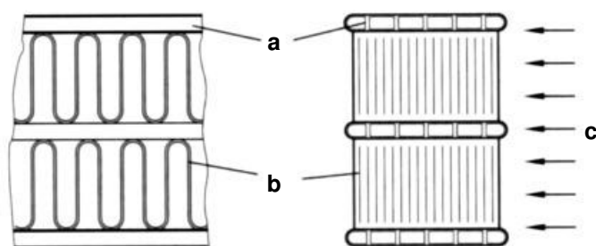
a Tube plat b Lamelles c Courant d'air
