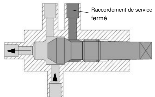
Tige de soupape complètement à droite (dans siège de retour)
