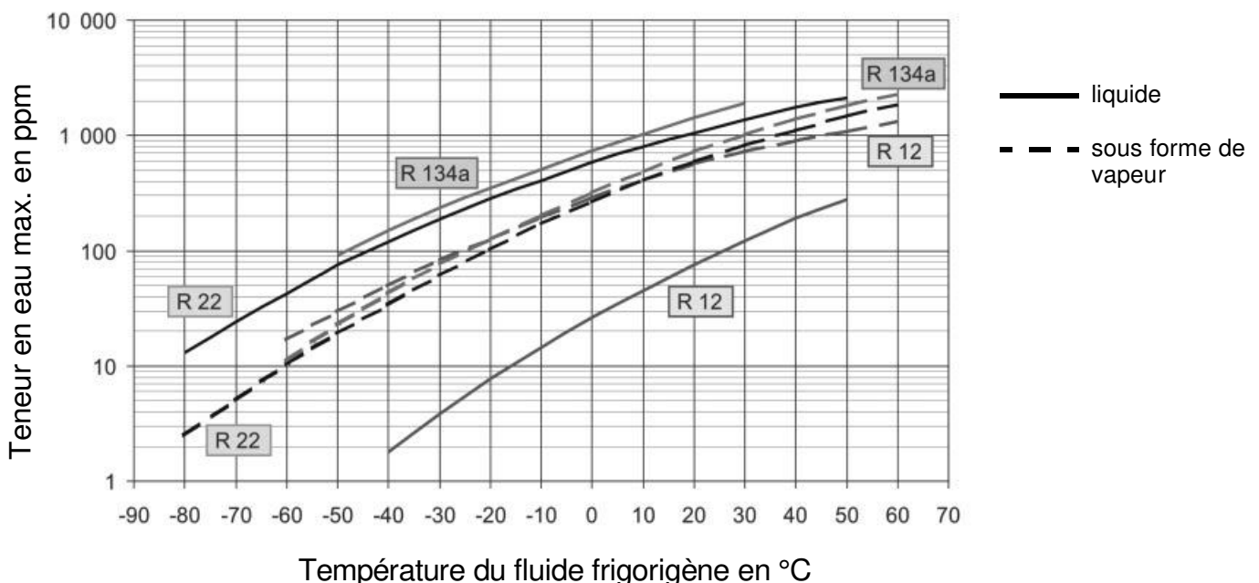
Fig 7-1. Teneur en eau maximale pour différents fluides frigorifiques
