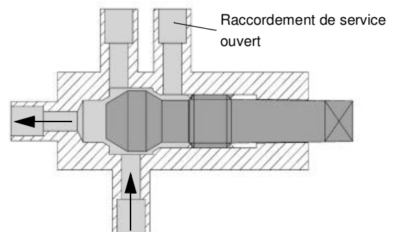
Tige de soupape complètement à droite (dans siège de retour)
